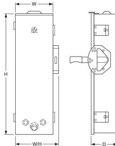
NEMA 3R
