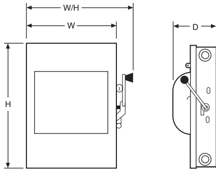
NEMA 1
