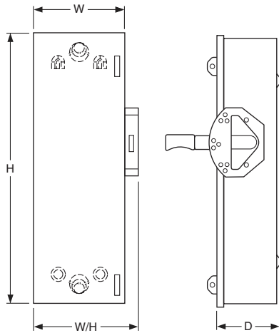
NEMA 1
